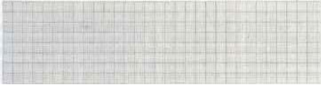
Şekil 1. EKG kağıdı
